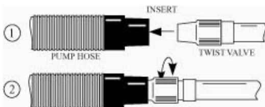
Ventil mit Drehverschluss (kein Adapter nötig) N° 1-3 + 6-7 Air Kanu
