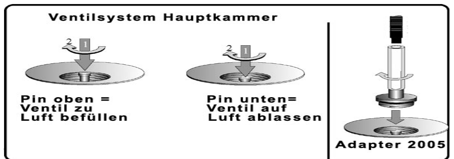
Ventilsystem Air Kanu u. Strait Edge Hauptkammer
